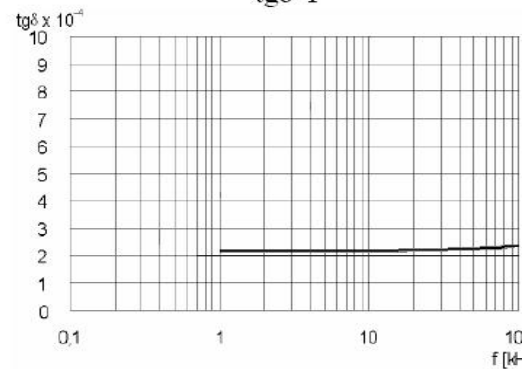
tg\delta -f
